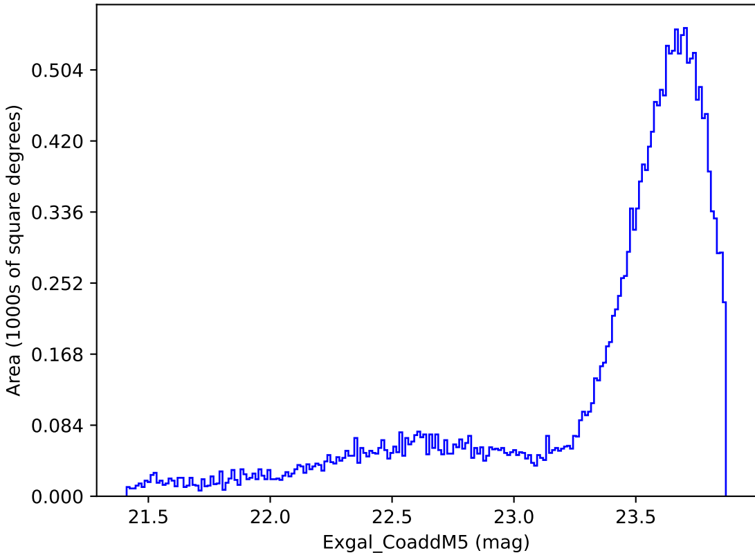
too_elab_r256_d3_ugrizy_v3.4_10yrs Yr 1 y band: Exgal_CoaddM5
