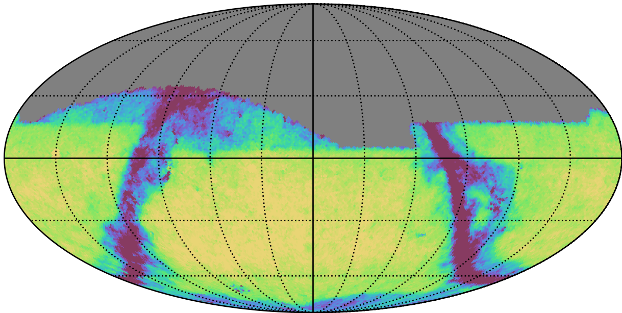
too_elab_r256_d3_ugrizy_v3.4_10yrs Yr 1 i band: Exgal_CoaddM5
