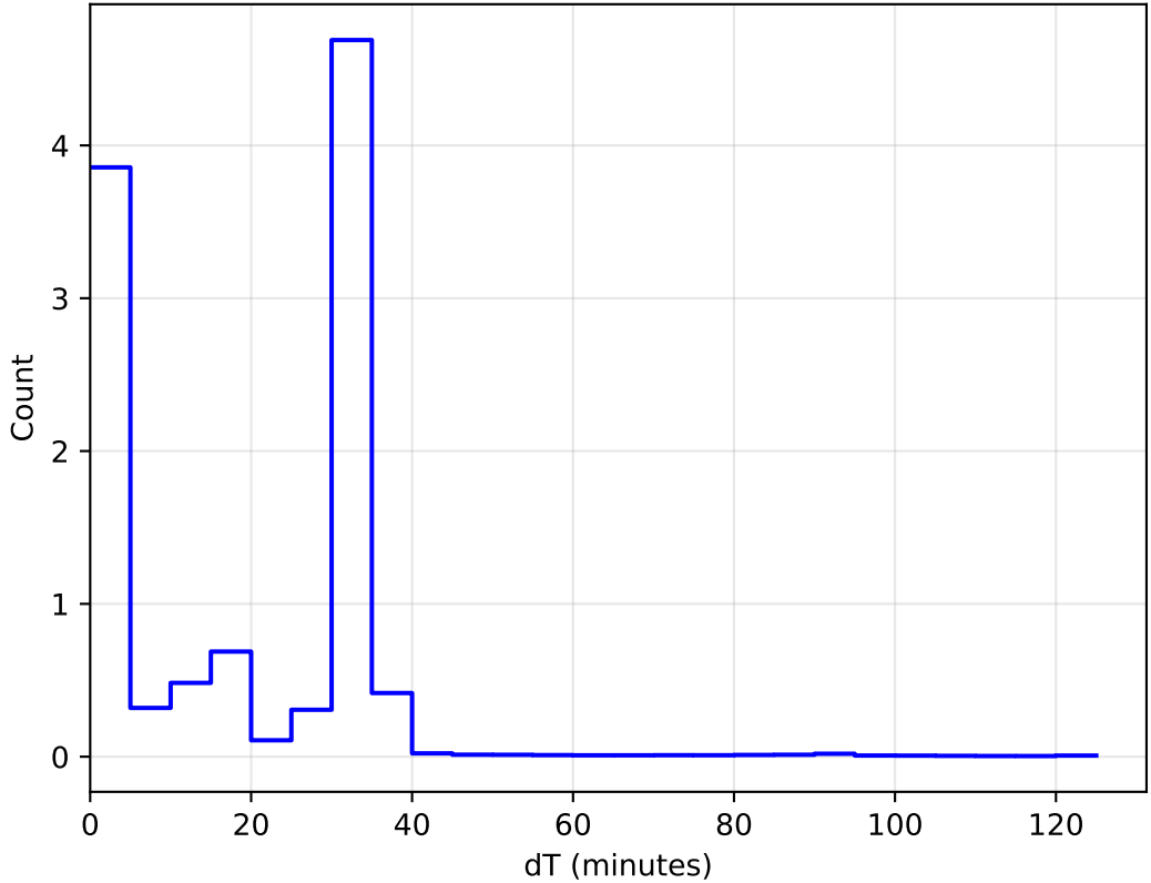
too_elab_r256_d3_ugrizy_v3.4_10yrs WFD: DeltaT Histogram 1e6
