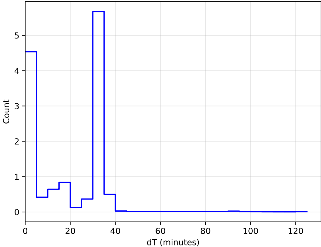
too_elab_r256_d3_ugrizy_v3.4_10yrs All sky: DeltaT Histogram 1e6
