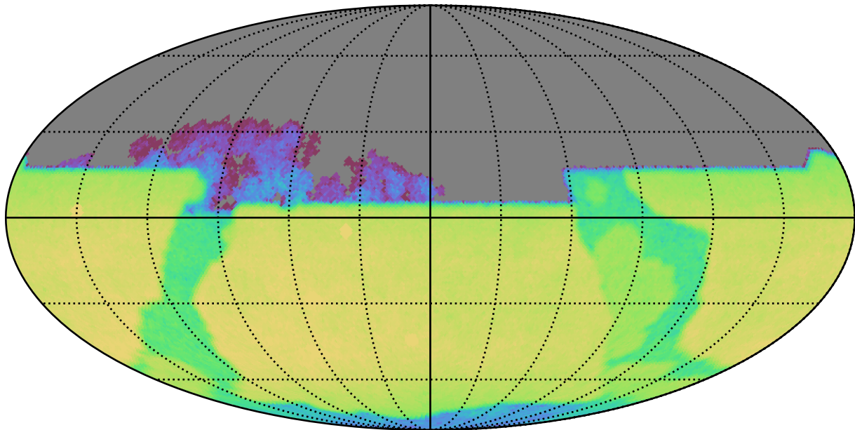
too_elab_r256_d3_ugrizy_v3.4_10yrs All sky y band: CoaddM5
