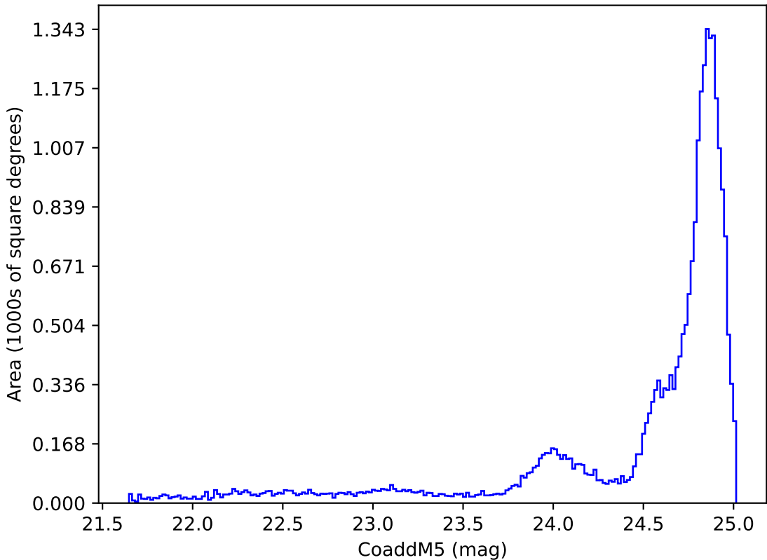
too_elab_r256_d3_ugrizy_v3.4_10yrs All sky y band: CoaddM5
