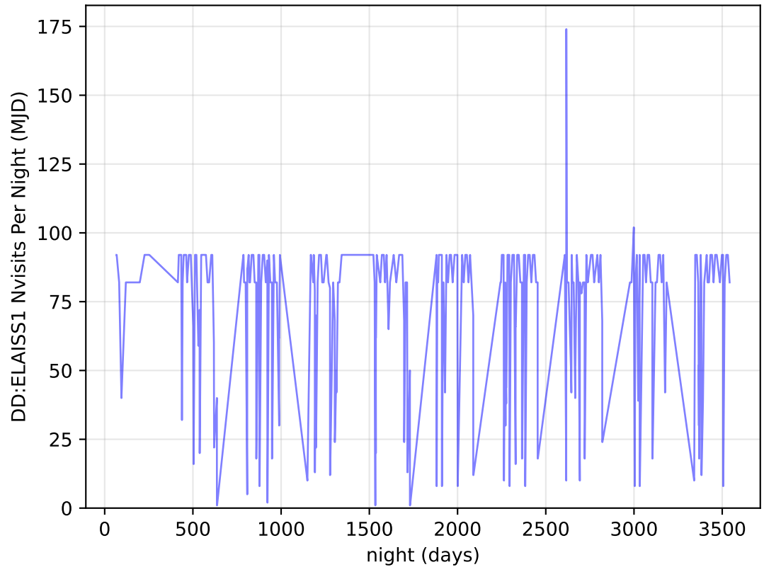
too_elab_r256_d3_ugrizy_v3.4_10yrs all bands: DD:ELAISS1 Nvisits Per Night
