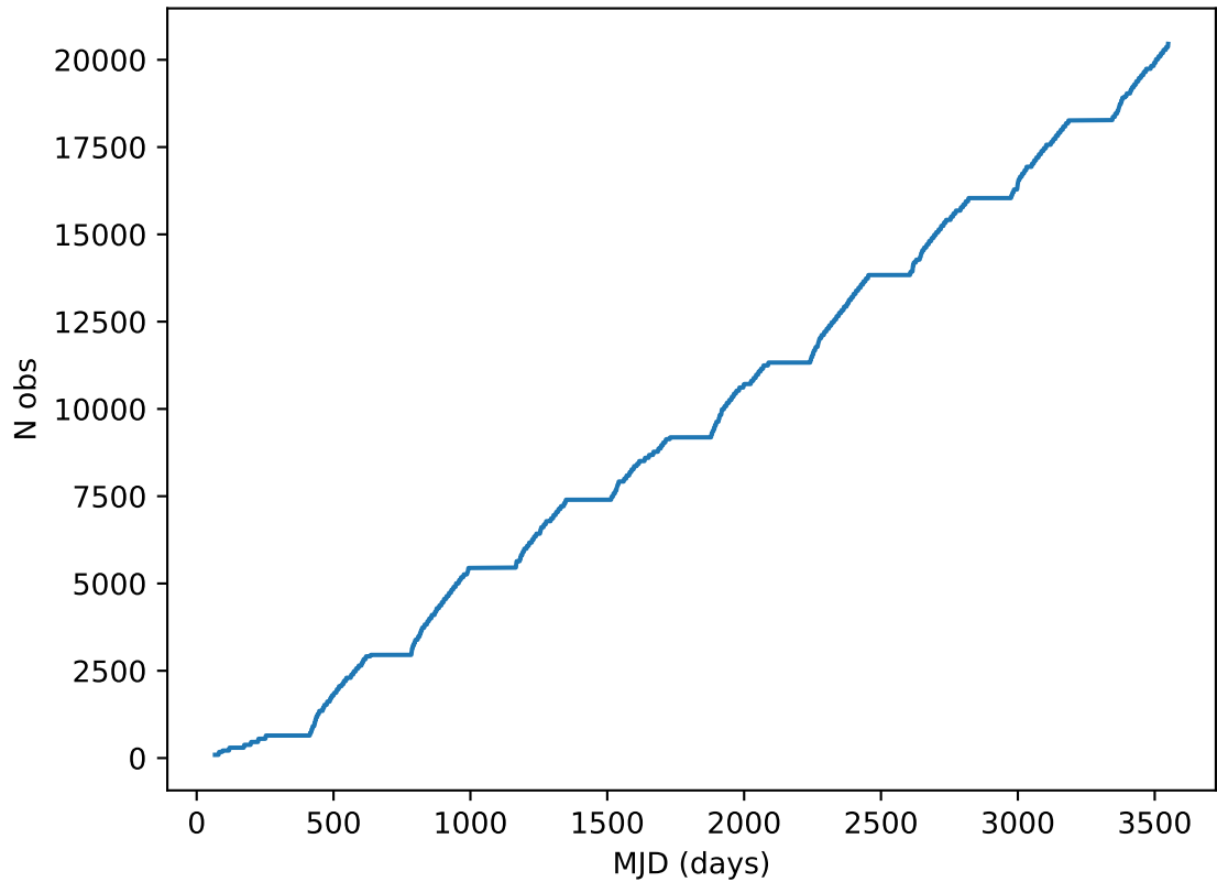
too_elab_r256_d3_ugrizy_v3.4_10yrs all bands: DD:ELAISS1 Cumulative NVisits
