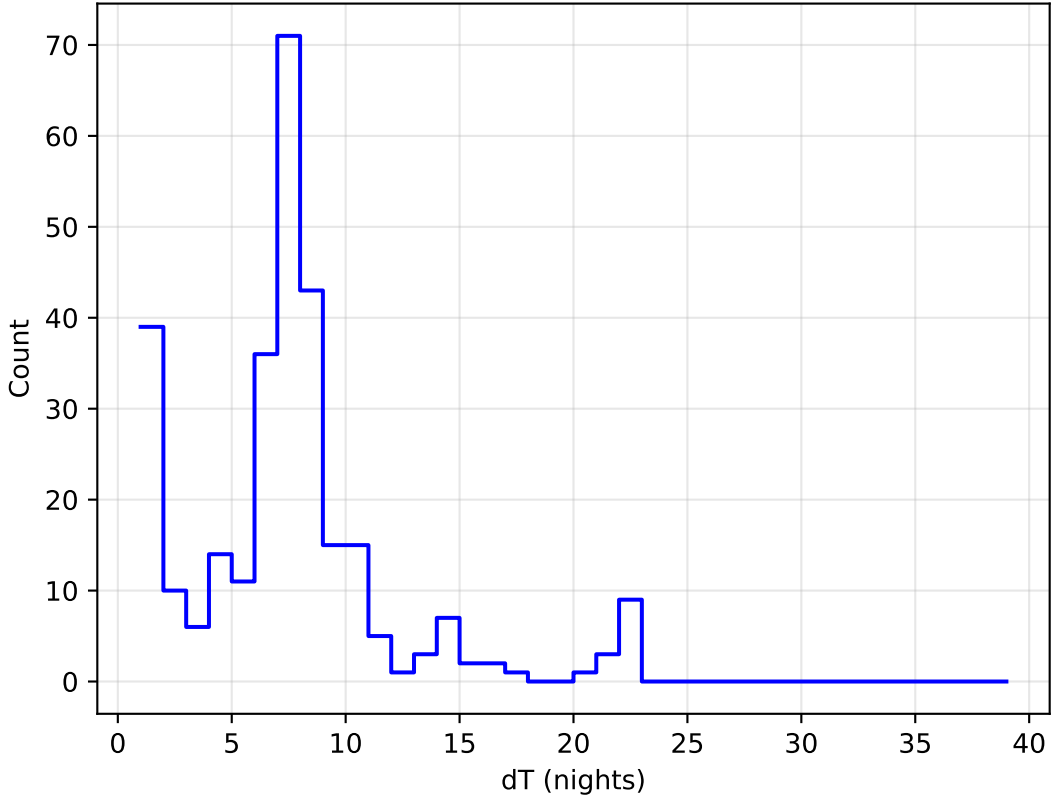
too_elab_r256_d3_ugrizy_v3.4_10yrs all bands: DD:EDFS Delta Nights Histogram
