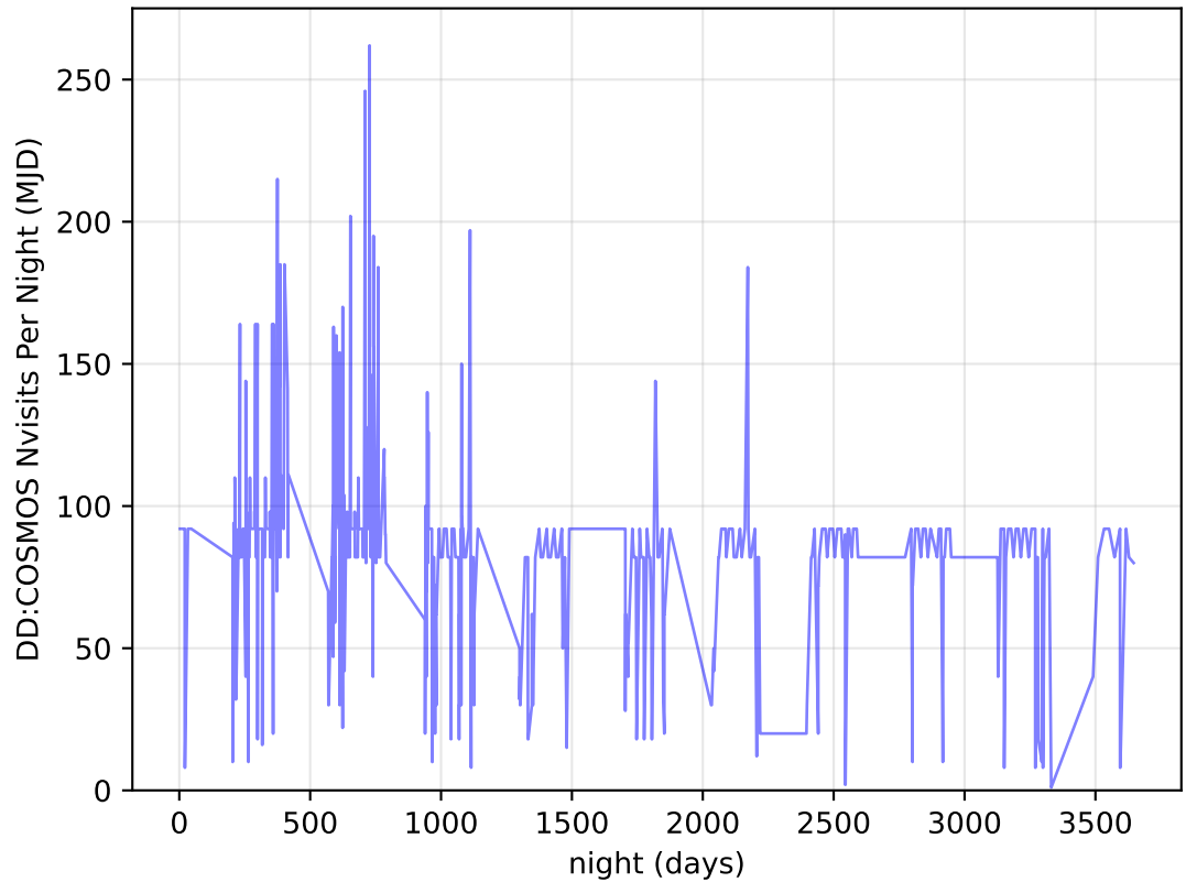
too_elab_r256_d3_ugrizy_v3.4_10yrs all bands: DD:COSMOS Nvisits Per Night
