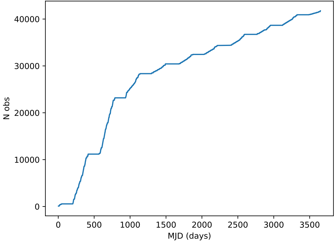
too_elab_r256_d3_ugrizy_v3.4_10yrs all bands: DD:COSMOS Cumulative NVisits
