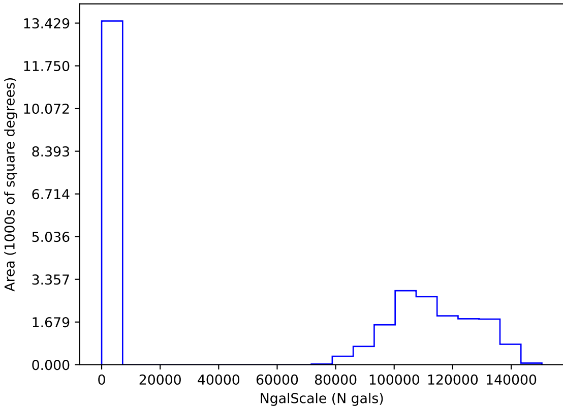
too_elab_r256_d3_gz_v3.4_10yrs i: NgalScale
