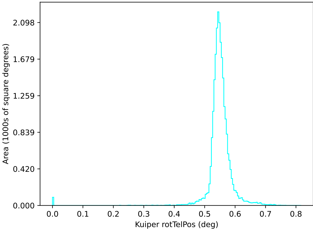
too_elab_r256_d3_gz_v3.4_10yrs u: Kuiper rotTelPos
