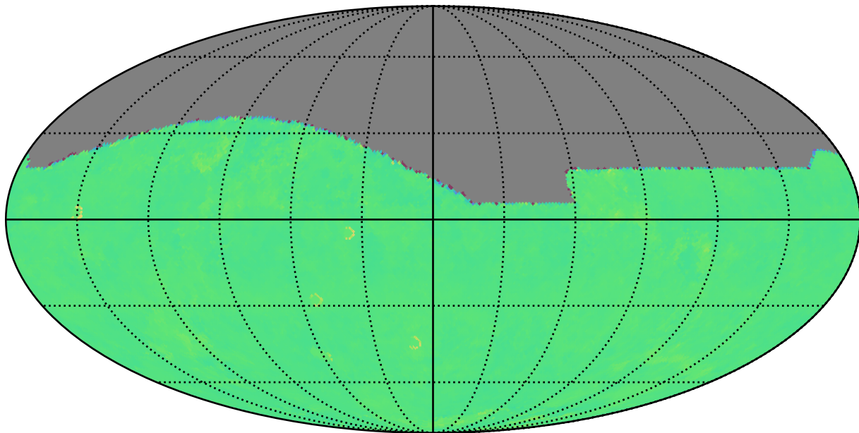
too_elab_r256_d3_gz_v3.4_10yrs i: Kuiper rotTelPos
