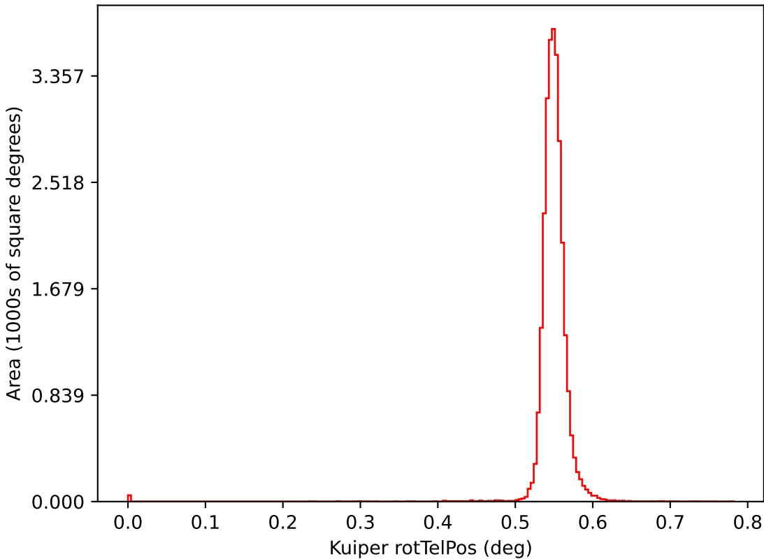
too_elab_r256_d3_gz_v3.4_10yrs i: Kuiper rotTelPos
