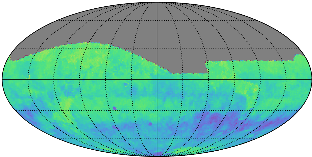
too_elab_r256_d3_gz_v3.4_10yrs i: Kuiper rotSkyPos
