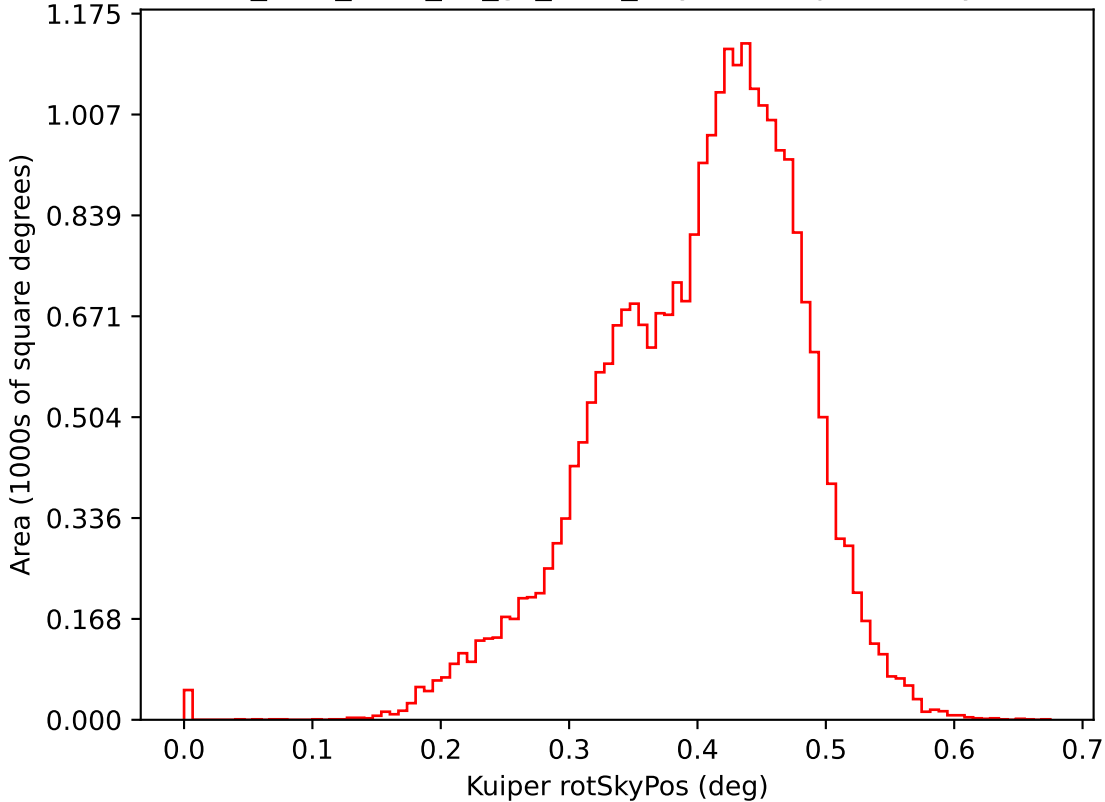
too_elab_r256_d3_gz_v3.4_10yrs i: Kuiper rotSkyPos
