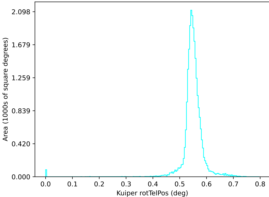
too_elab_r256_d3_griz_v3.4_10yrs u: Kuiper rotTelPos
