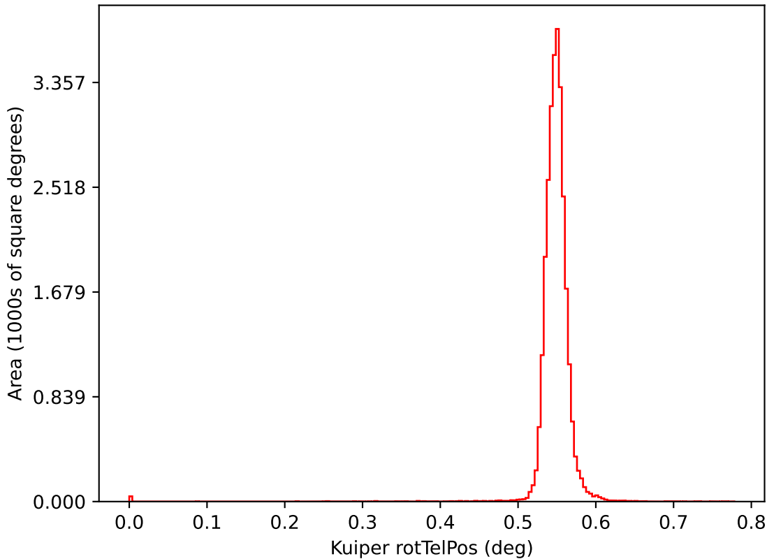
too_elab_r256_d3_griz_v3.4_10yrs i: Kuiper rotTelPos
