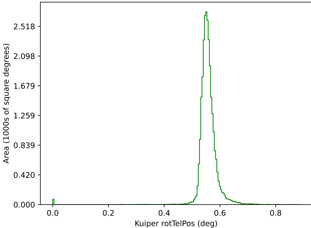
too_elab_r256_d3_griz_v3.4_10yrs g: Kuiper rotTelPos
