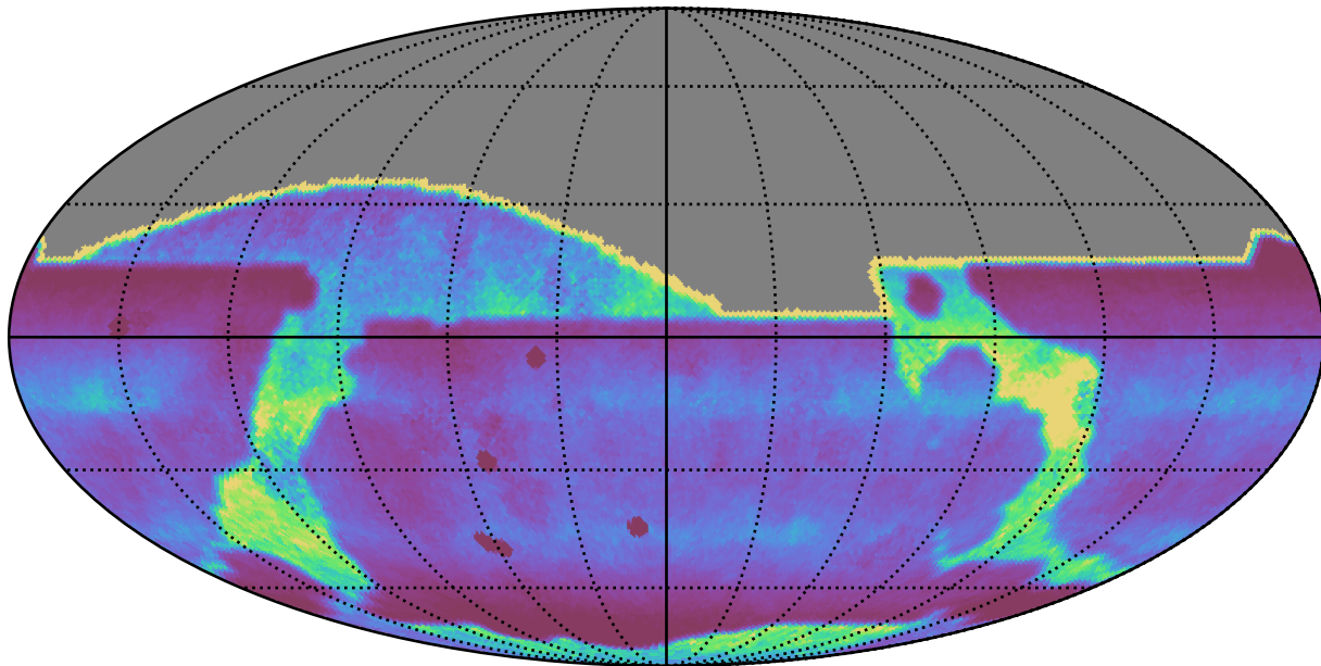
too_elab_r256_d3_griz_v3.4_10yrs : DCRprecision
