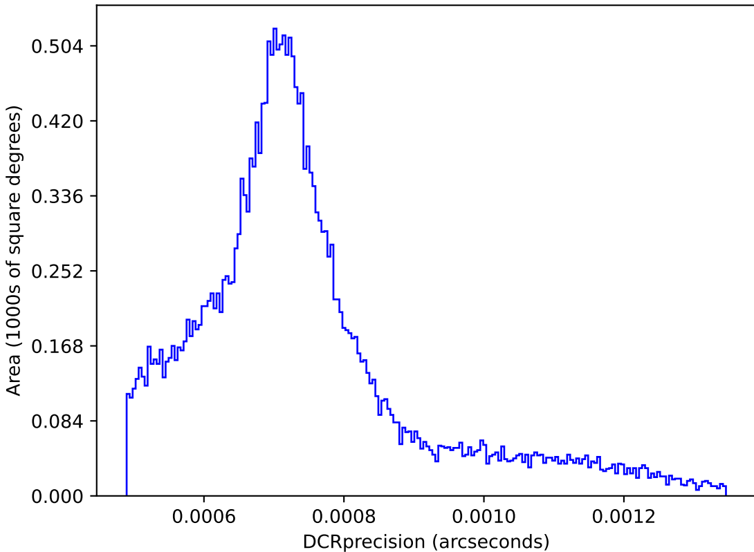
too_elab_r256_d3_griz_v3.4_10yrs : DCRprecision
