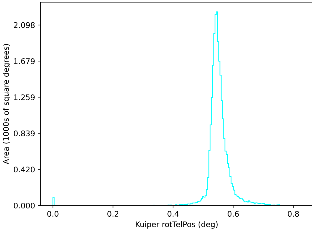
too_elab_r256_d3_giz_v3.4_10yrs u: Kuiper rotTelPos
