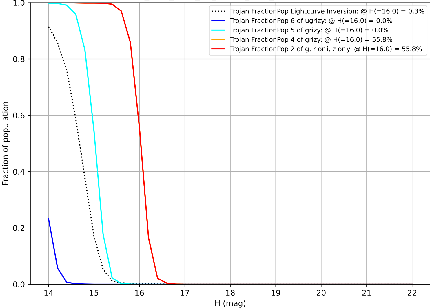
too_elab_r256_d2_ugrizy_v3.4_10yrs Trojan
