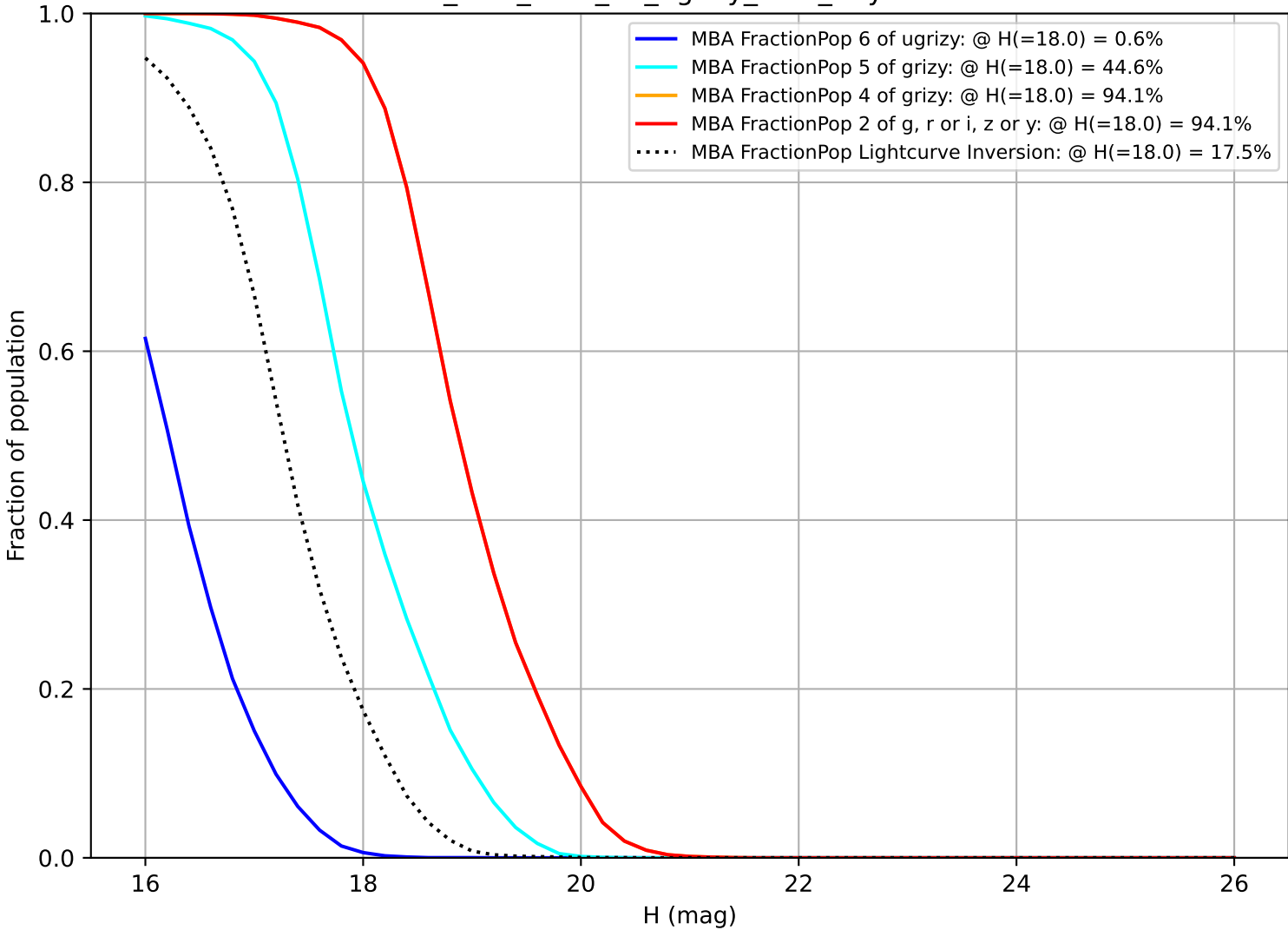
too_elab_r256_d2_ugrizy_v3.4_10yrs MBA
