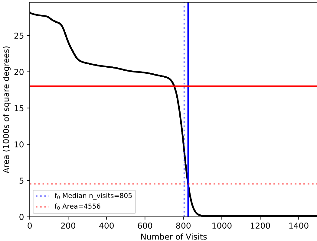
too_elab_r256_d2_ugrizy_v3.4_10yrs : f0
