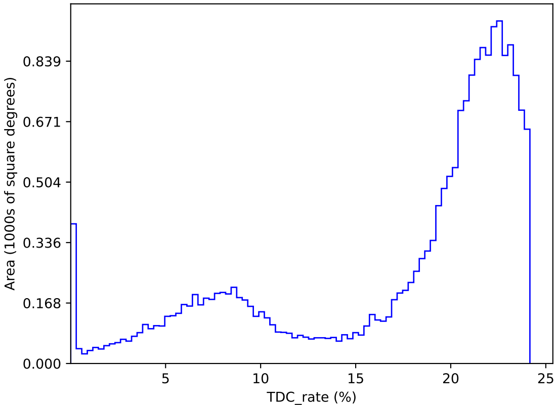
too_elab_r256_d2_ugrizy_v3.4_10yrs : TDC_rate
