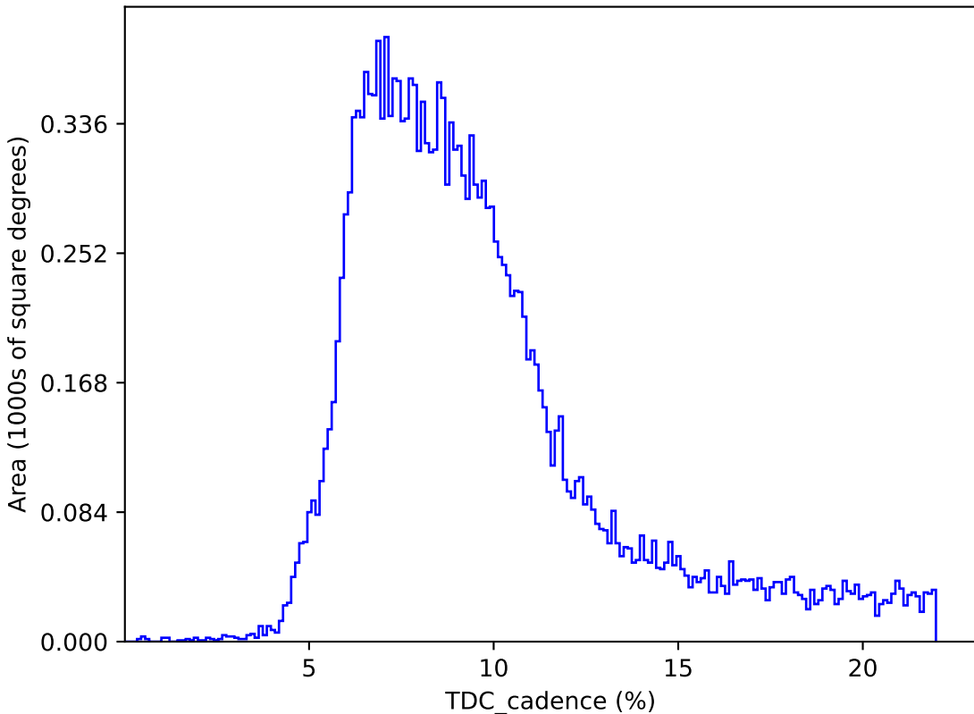
too_elab_r256_d2_ugrizy_v3.4_10yrs : TDC_cadence
