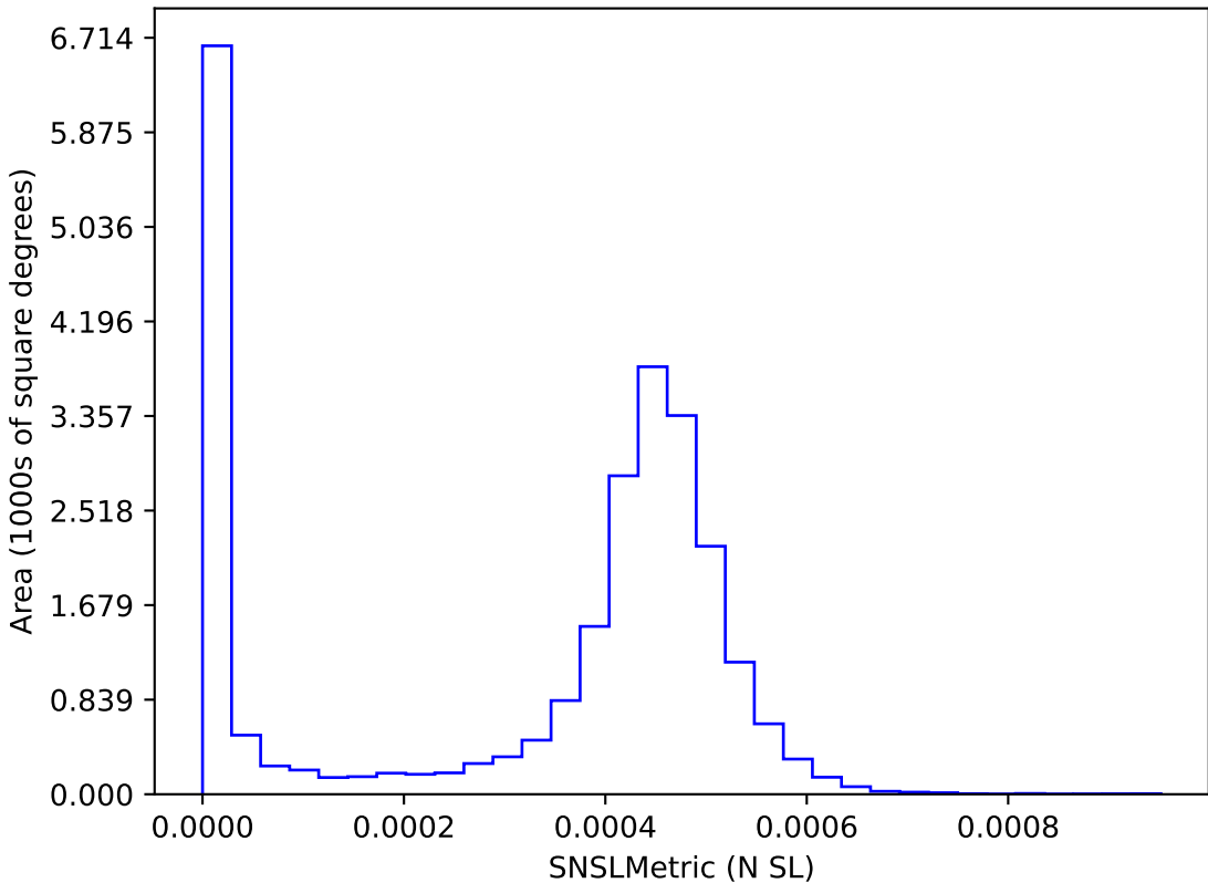
too_elab_r256_d2_ugrizy_v3.4_10yrs : SNSLMetric
