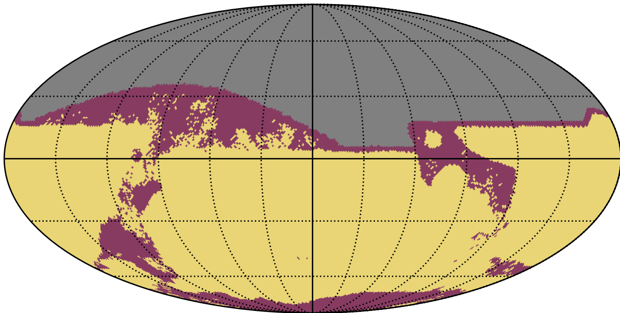
too_elab_r256_d2_ugrizy_v3.4_10yrs : RapidRevisits
