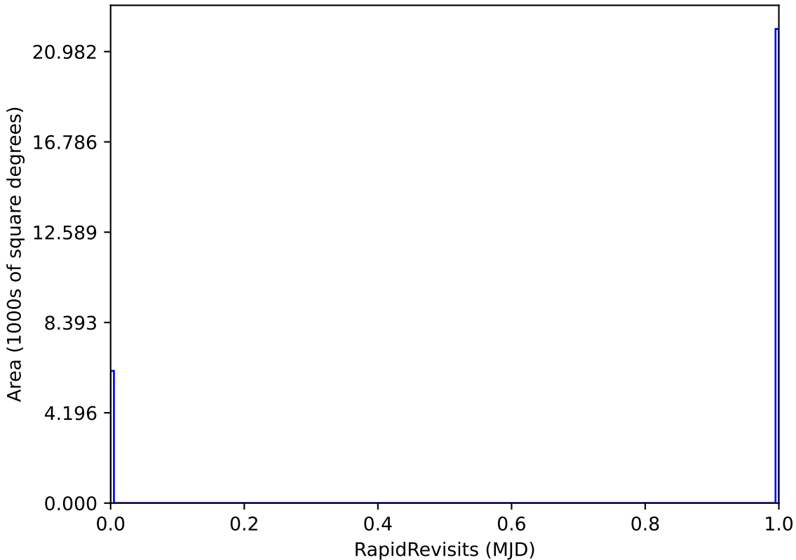
too_elab_r256_d2_ugrizy_v3.4_10yrs : RapidRevisits
