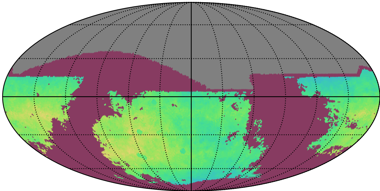
too_elab_r256_d2_ugrizy_v3.4_10yrs i: NgalScale
