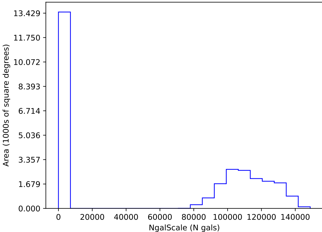
too_elab_r256_d2_ugrizy_v3.4_10yrs i: NgalScale
