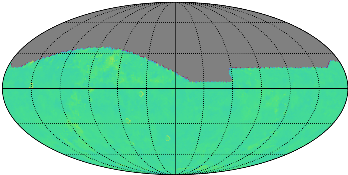
too_elab_r256_d2_ugrizy_v3.4_10yrs z: Kuiper rotTelPos
