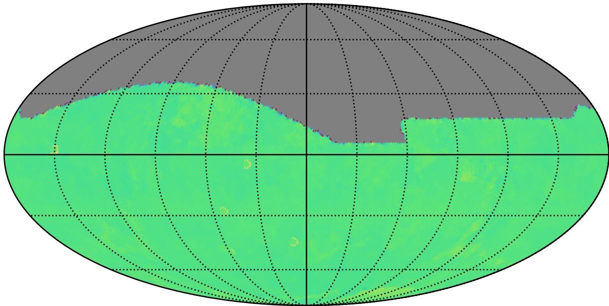
too_elab_r256_d2_ugrizy_v3.4_10yrs r: Kuiper rotTelPos
