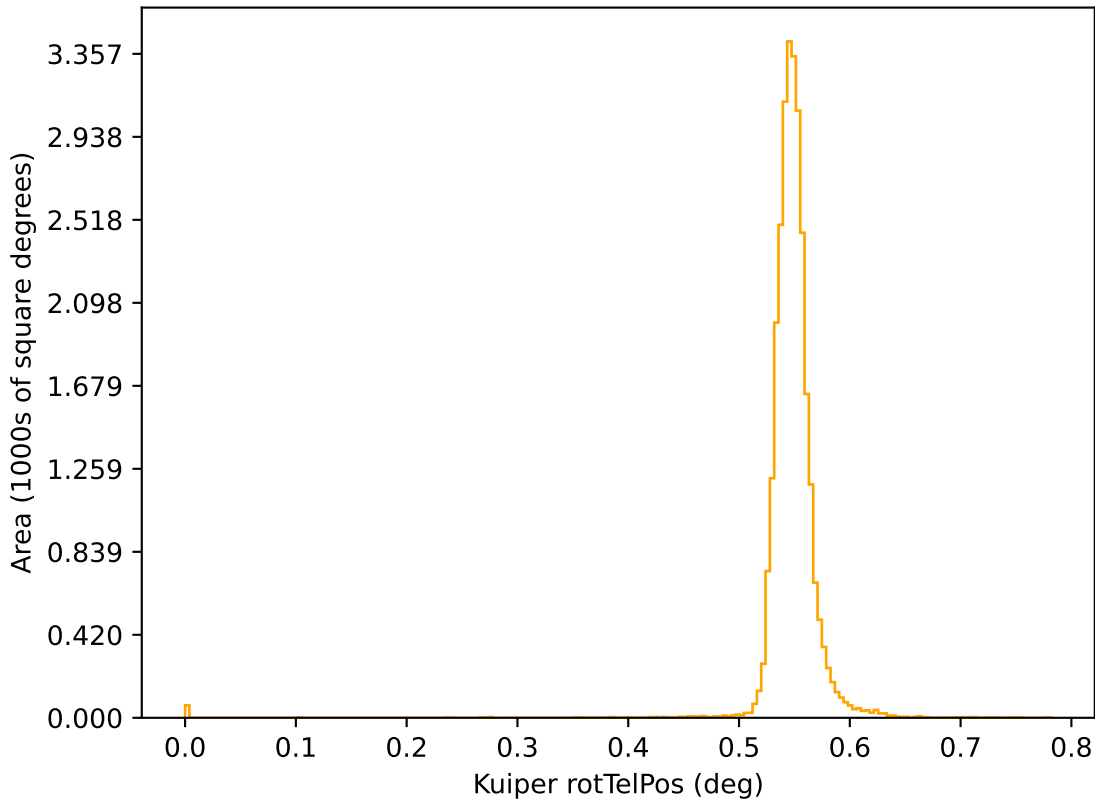
too_elab_r256_d2_ugrizy_v3.4_10yrs r: Kuiper rotTelPos
