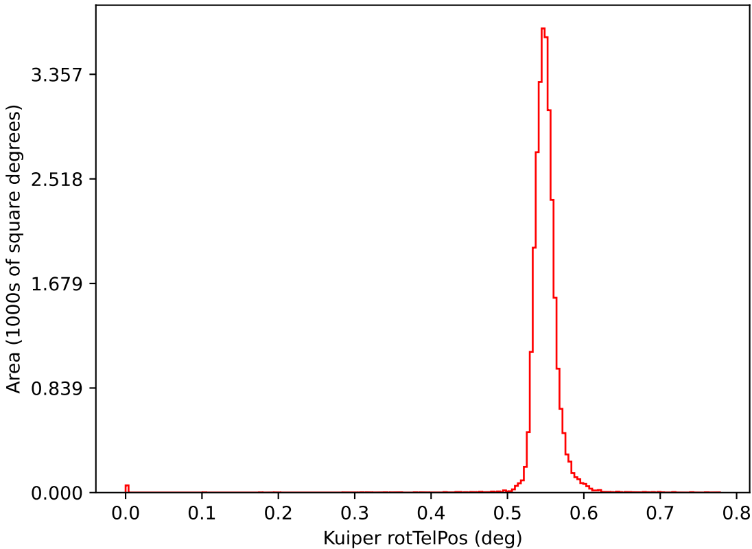
too_elab_r256_d2_ugrizy_v3.4_10yrs i: Kuiper rotTelPos
