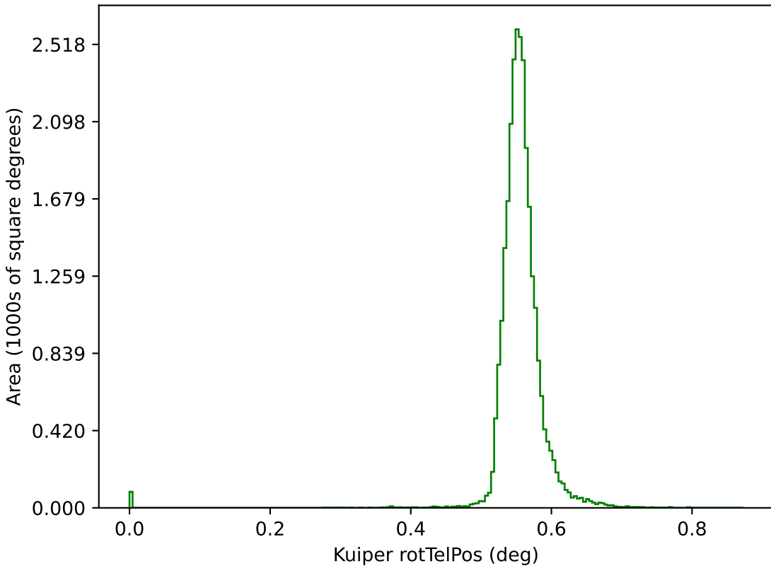
too_elab_r256_d2_ugrizy_v3.4_10yrs g: Kuiper rotTelPos
