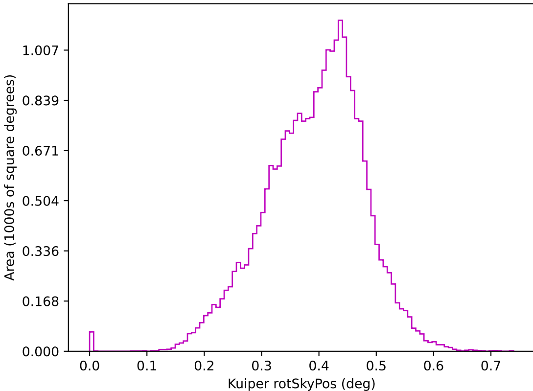
too_elab_r256_d2_ugrizy_v3.4_10yrs z: Kuiper rotSkyPos
