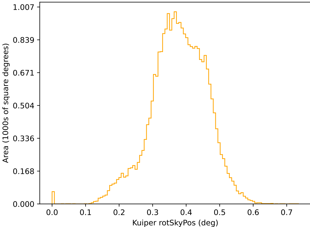
too_elab_r256_d2_ugrizy_v3.4_10yrs r: Kuiper rotSkyPos
