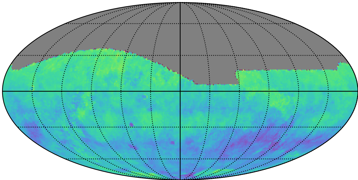
too_elab_r256_d2_ugrizy_v3.4_10yrs i: Kuiper rotSkyPos
