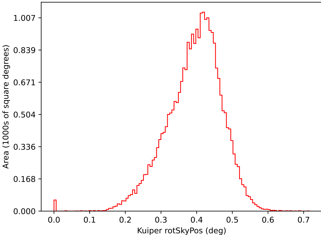
too_elab_r256_d2_ugrizy_v3.4_10yrs i: Kuiper rotSkyPos
