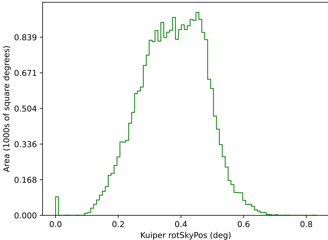
too_elab_r256_d2_ugrizy_v3.4_10yrs g: Kuiper rotSkyPos
