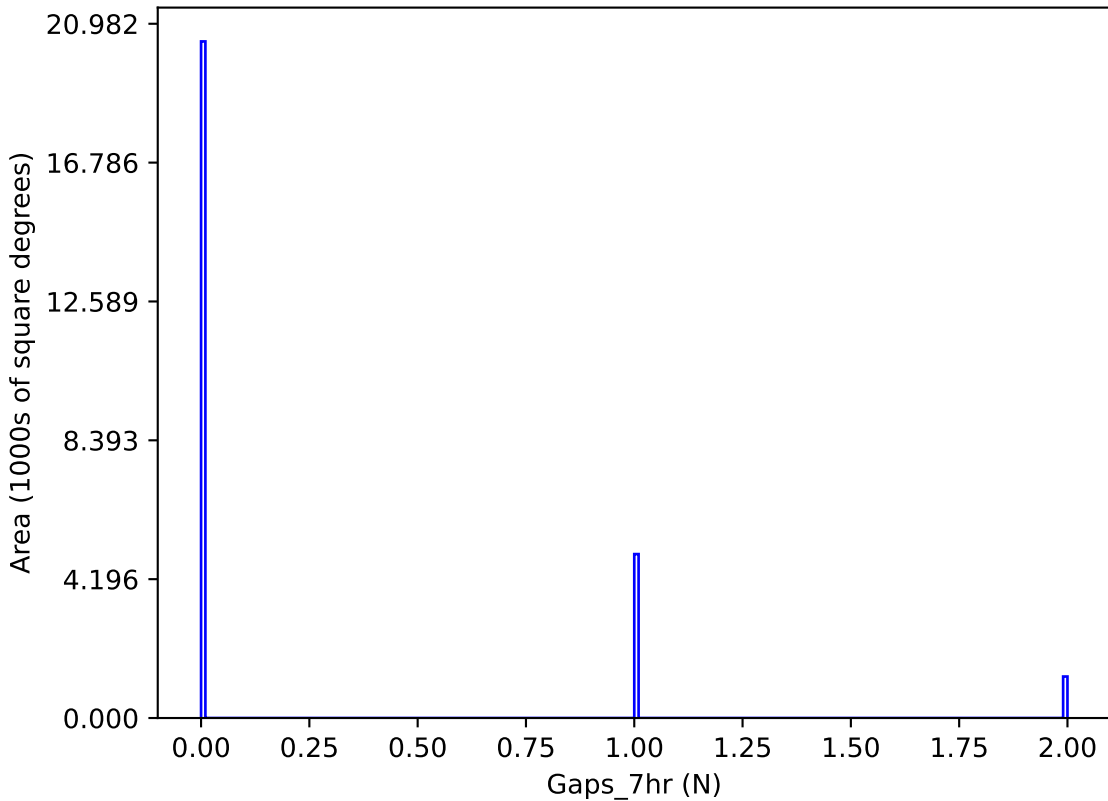
too_elab_r256_d2_ugrizy_v3.4_10yrs y band: Gaps_7hr
