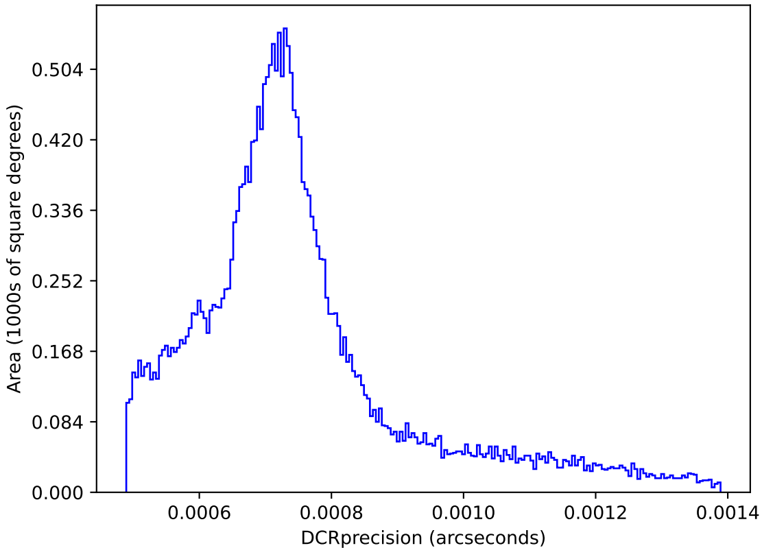
too_elab_r256_d2_ugrizy_v3.4_10yrs : DCRprecision
