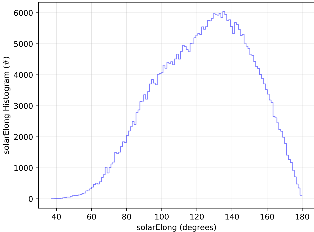
too_elab_r256_d2_ugrizy_v3.4_10yrs WFD y band: solarElong Histogram
