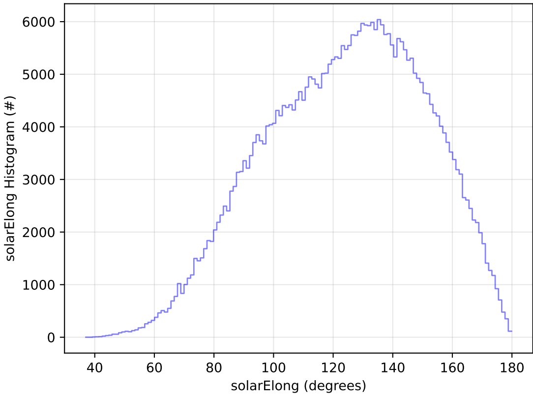
too_elab_r256_d2_ugrizy_v3.4_10yrs All sky y band: solarElong Histogram
