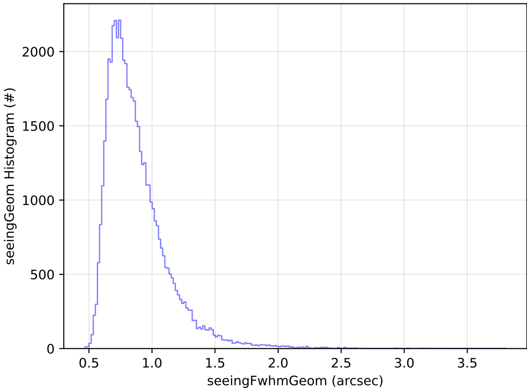
too_elab_r256_d2_ugrizy_v3.4_10yrs Yr 1 i band: seeingGeom Histogram
