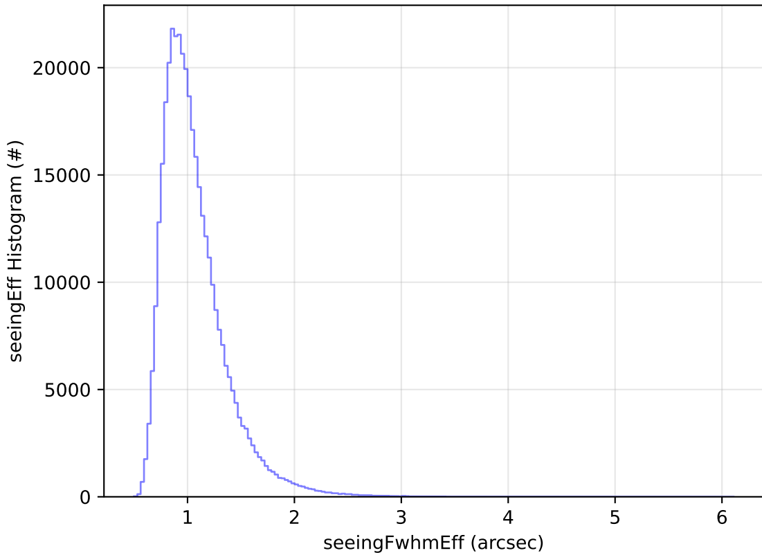
too_elab_r256_d2_ugrizy_v3.4_10yrs WFD y band: seeingEff Histogram
