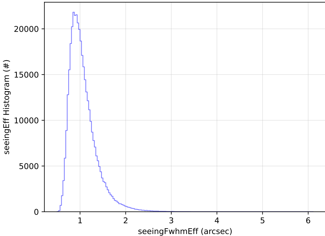
too_elab_r256_d2_ugrizy_v3.4_10yrs All sky y band: seeingEff Histogram
